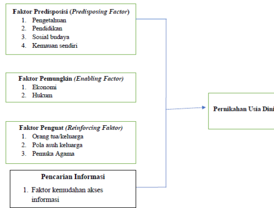
Gambar. 1 Kerangka Berfikir
